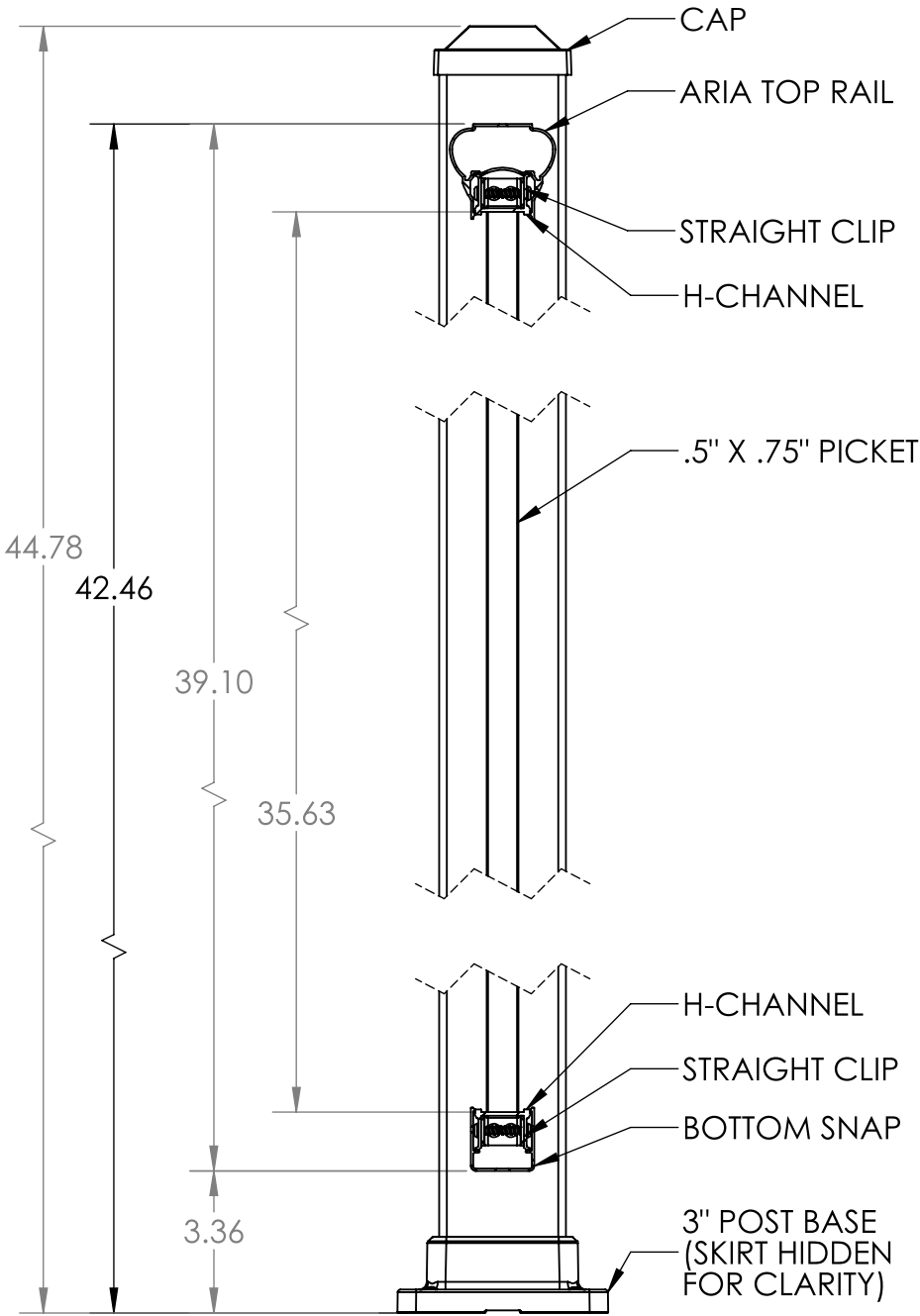
SECTION A-A
